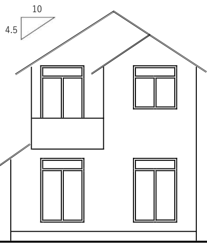
南側立面図
